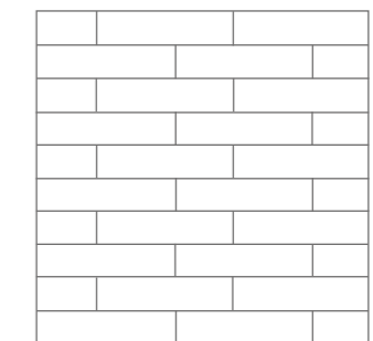
ENGLISCHER VERBAND
